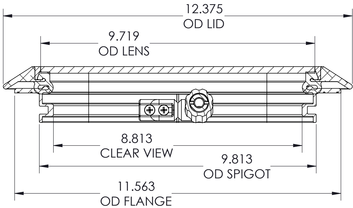
SECTION A-A
